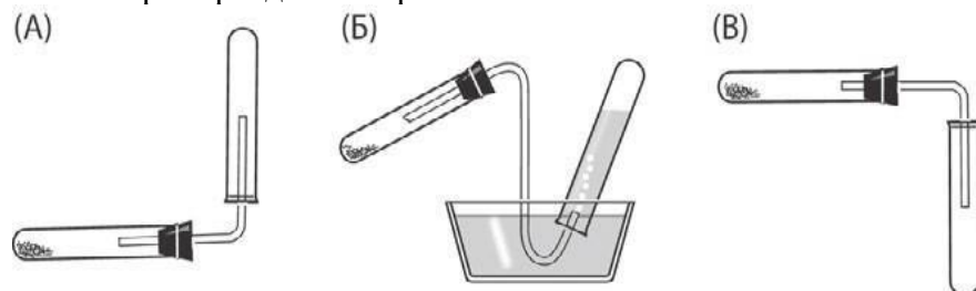
Рис. 7. Приборы для собирания газов
